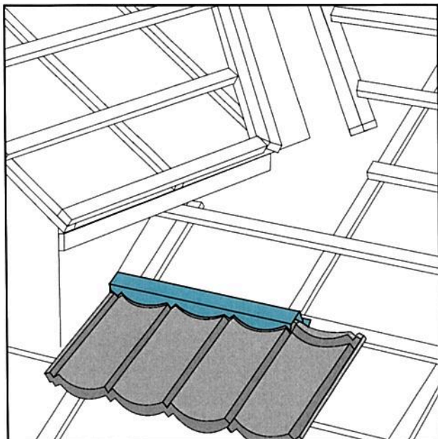
1. Z-profilen tilpasses på lengden slik at den avsluttes på en bølgetopp.
