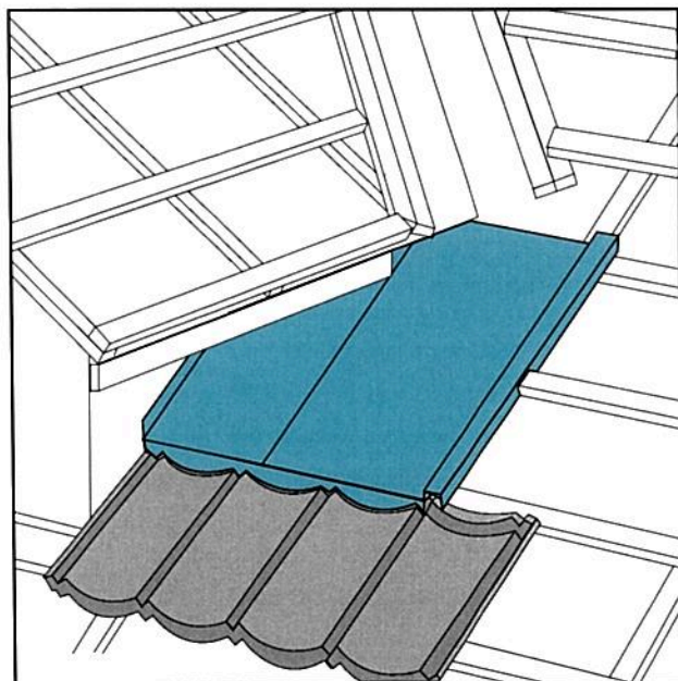
3. Denne platen tilpasses med lik lengde som foregående plate. Platene skal nå ligge med overlapp og skrues deretter fast i z-profilen under.
